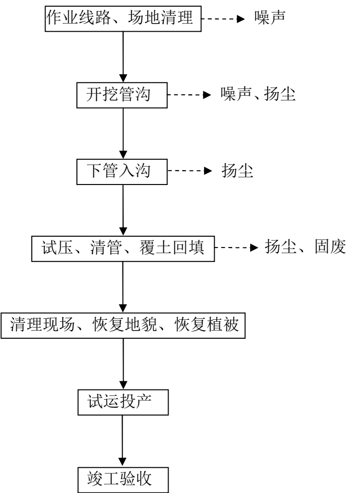
图 6-1 污水管网施工工艺流程图及产污环节图
